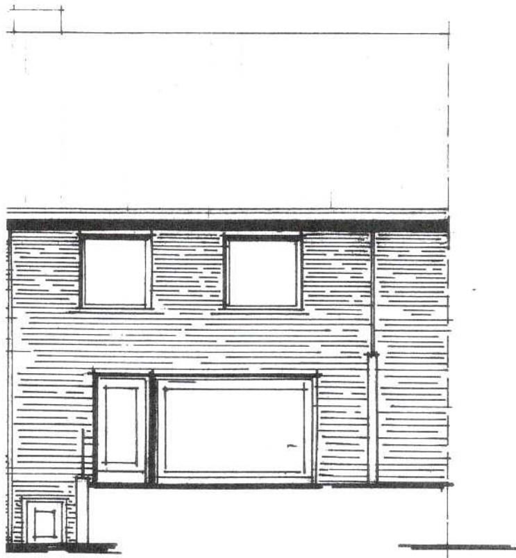
WESTANSICHT
