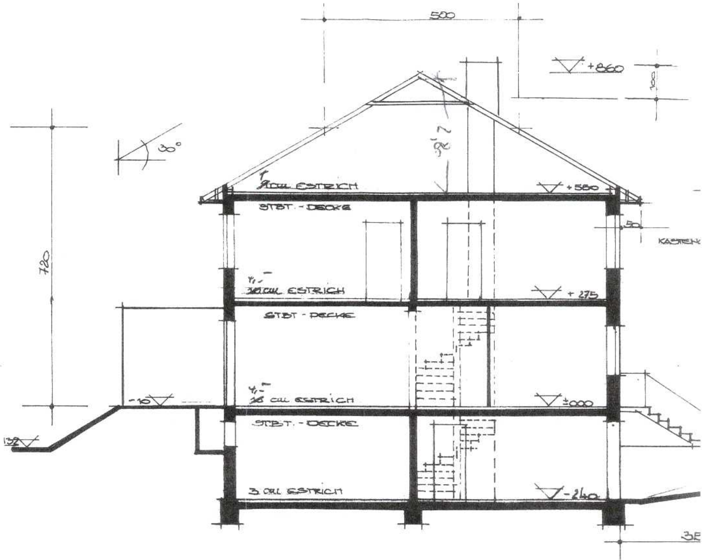
SCHNITT A-B
